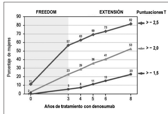
Figura 1. Porcentaje de mujeres que alcanzan una determinada puntuación T en columna lumbar y cadera total
